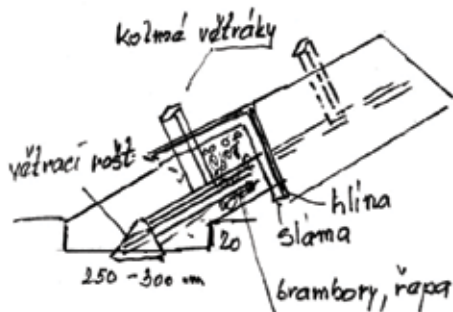
Nákres krechtu na uskladnění brambor a řepy.
